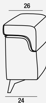
BRAZO PARA MÓDULOS (DE SERIE)
